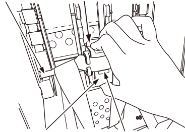
肩ハーネスアジャスター解除ボタン 緑色のラベル
