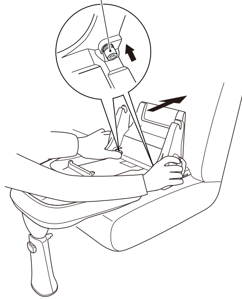
コネクター調整ボタン
